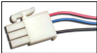
PN # TF-LRA25B50-01 24 Volt Replacement Fan for A25B50 Rectifier Unit (Lorain / Marconi) w/ 3 Wire Plug
