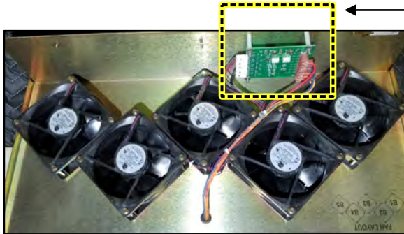
DMS-100 (NT3X90AF) FAN TRAY
