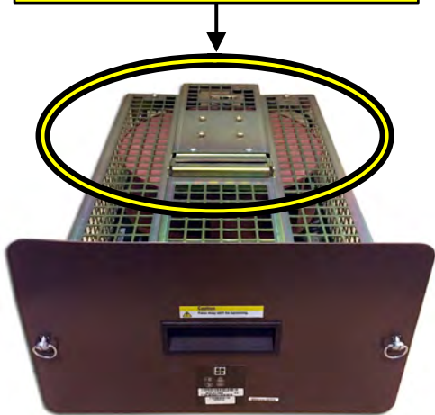
Existing 225mm Impeller Fan
