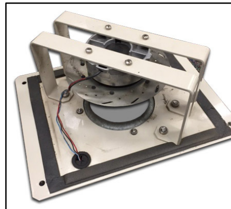
BROKEN FAN SHOWN (SINGLE FAN HOUSING)
